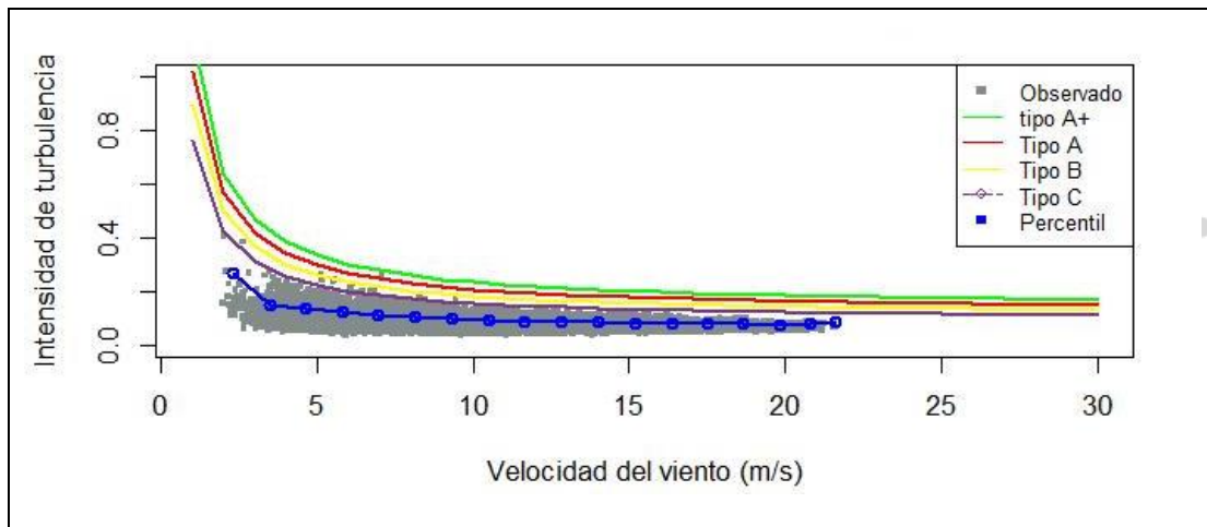
Figura 2. Intensidad de turbulencia vs Velocidad de viento según la norma IEC61400-1.
