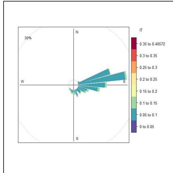
Figura 3. Rosa de intensidad de turbulencia.
