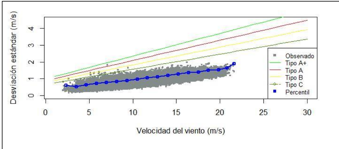
Figura 1. Desviación estándar vs Velocidad de viento según la norma IEC61400-1.
